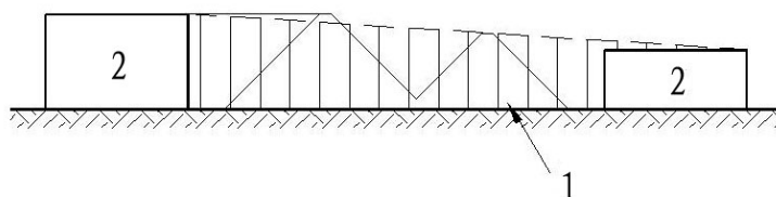
图 5.4.2-1 一字形防护土堤水平地形剖面防护范围 1—防护土堤有效防护范围；2—危险性建筑物
