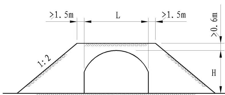
图 8.9.4 覆土库的覆土剖面示意图
