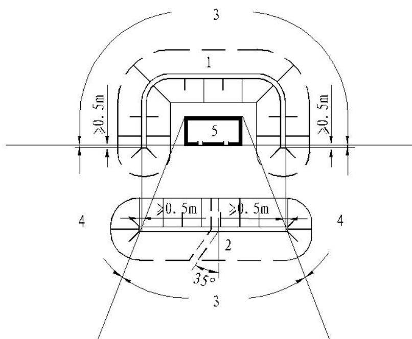
图 5.4.1-1 标准防护土堤的平面防护范围 1-II形防护土堤；2-I字形防护土堤；3-防护土堤有效防护范围 4-防护土堤无防护范围；5-危险性建筑物
